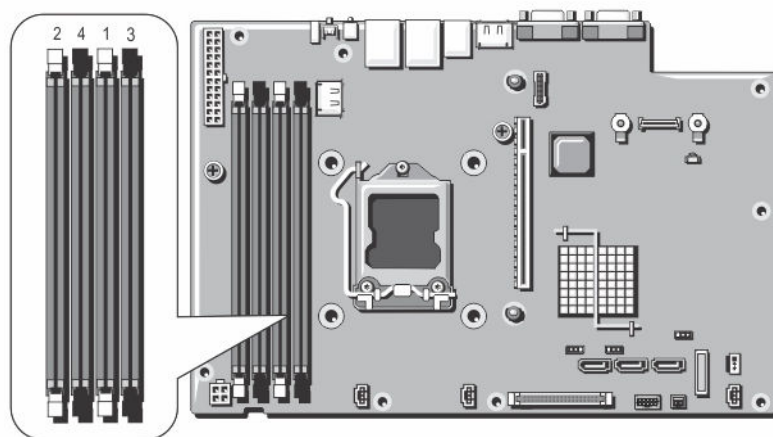
図 14. メモリソケットの位置
