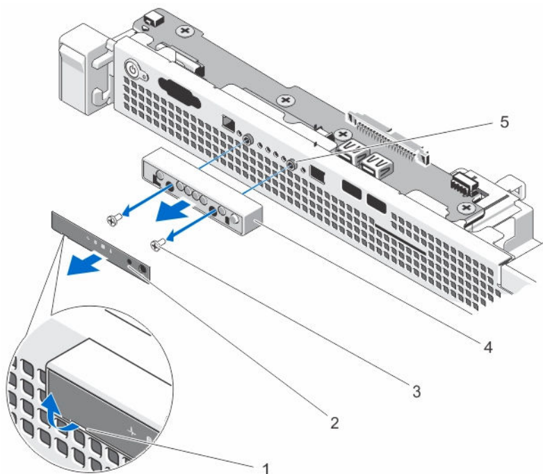
図 10. LED モジュールの取り外しと取り付け
