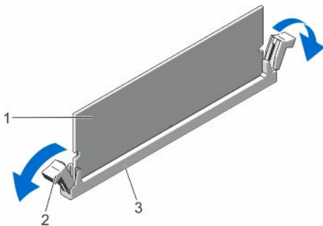
図 15. メモリモジュールの取り外し
