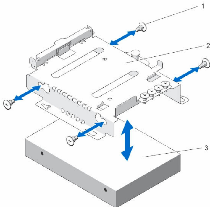
図 9. ハードドライブケースからの 3.5 インチハードドライブの取り外しと取り付け
