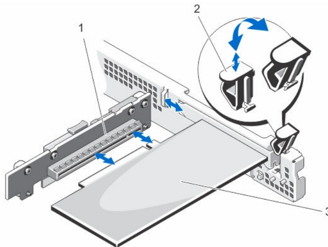
図 17. ライザーでの PERC h310 カードの取り外しと取り付け
