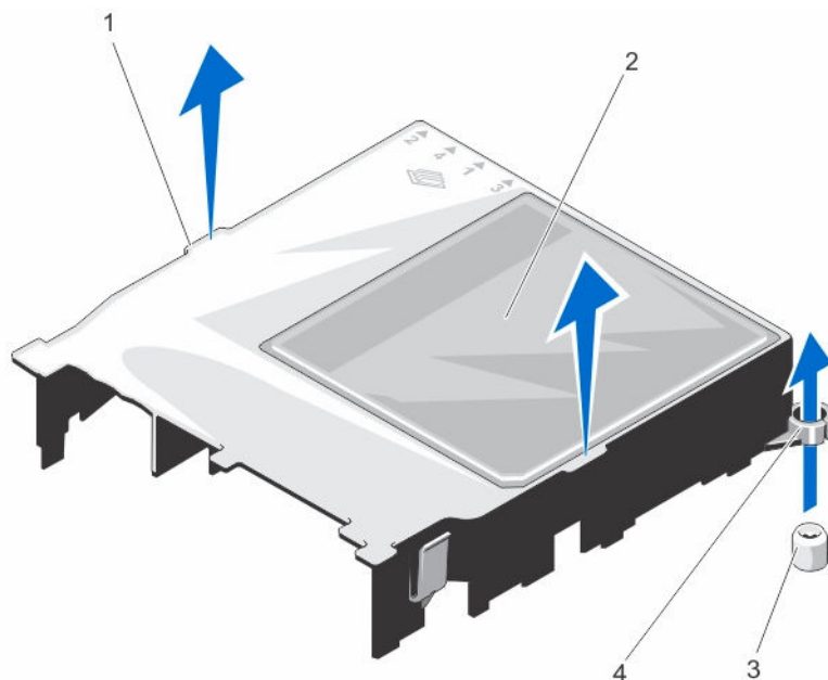
図 13. 冷却エアフローカバーの取り外しと取り付け
