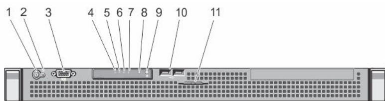
図 1. 前面パネルの機能とインジケータ
