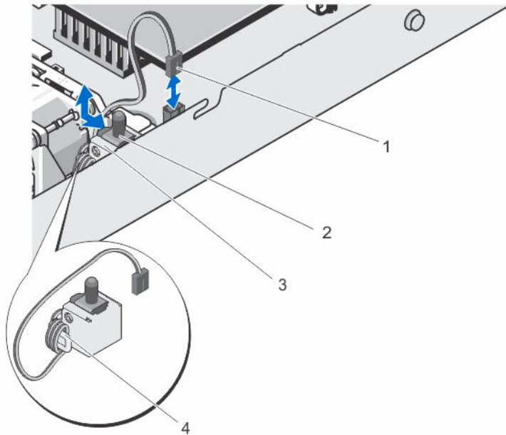
図7. シャーシイントルージョンスイッチの取り外しと取り付け
