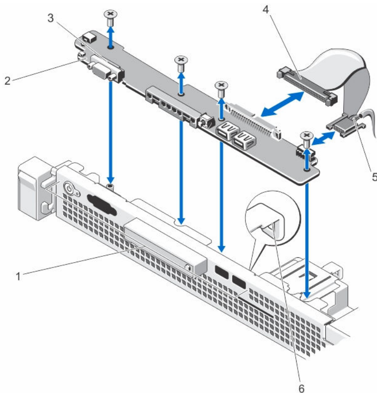
図 11. コントロールパネルボードの取り外しと取り付け
