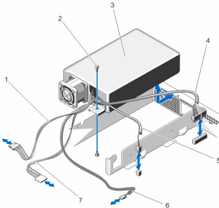
図 22. 電源装置ユニットの取り外しと取り付け
