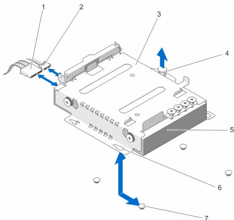
図 8. 3.5 インチハードドライブ (hdd1) ケージの取り外しと取り付け
