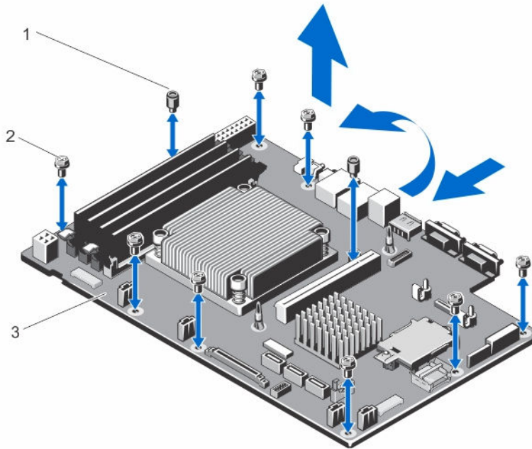
図 23. システム基板の取り外しと取り付け
