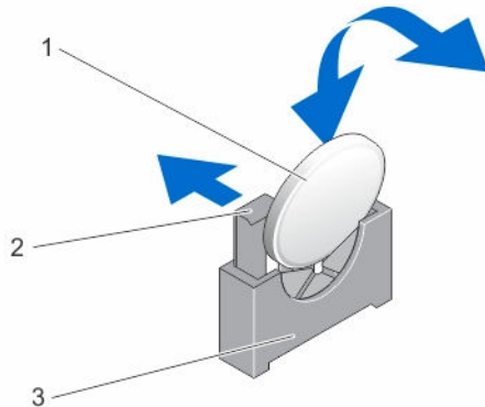
図 19. システムバッテリーの交換
